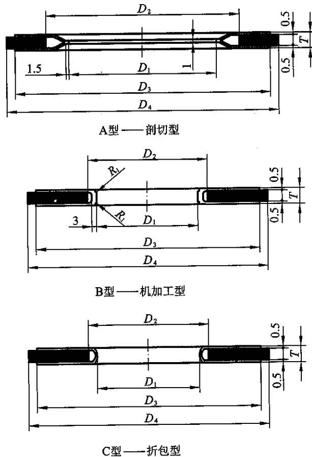
图 3.0.1 垫片的型式
