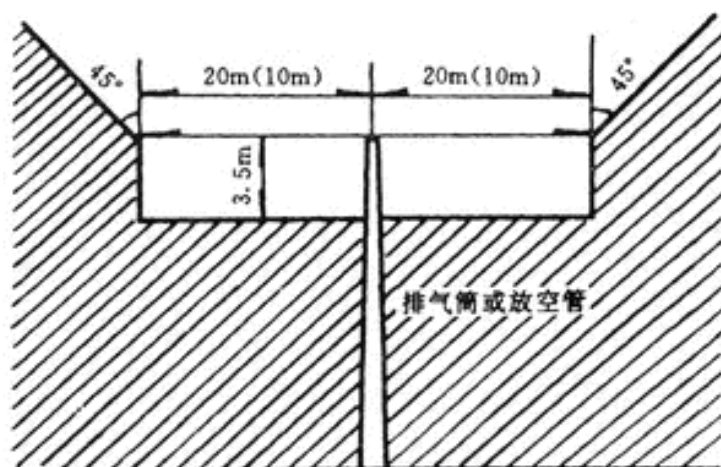
图5.5.11 可燃气体的排气筒、放空管高度示意图
