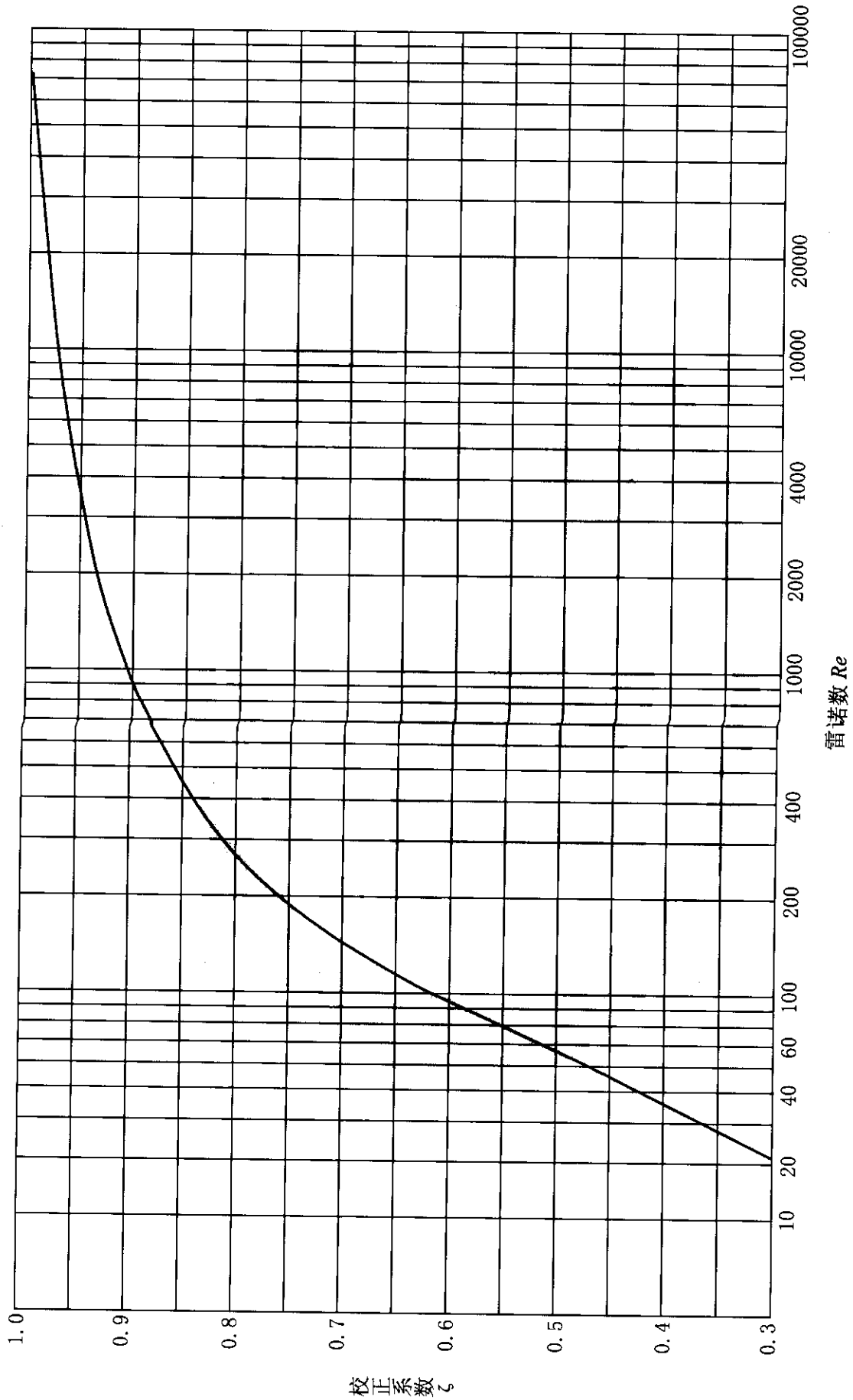
图 E-2 液体动力粘度校正系数 \zeta
