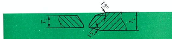
图 8.2.5-3 内外壁均不齐平不同壁厚管道组成件坡口侧加工
