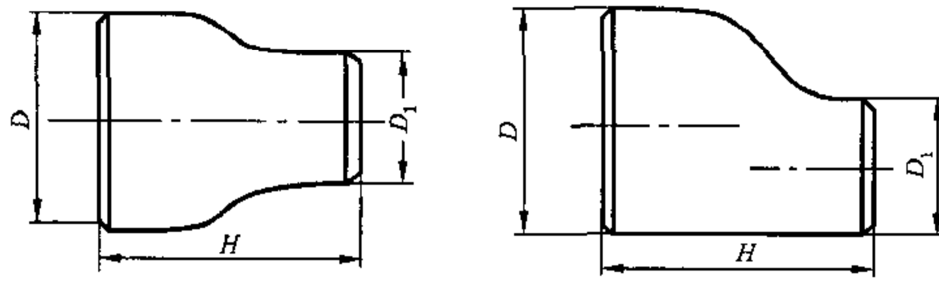
图 10 异径接头
