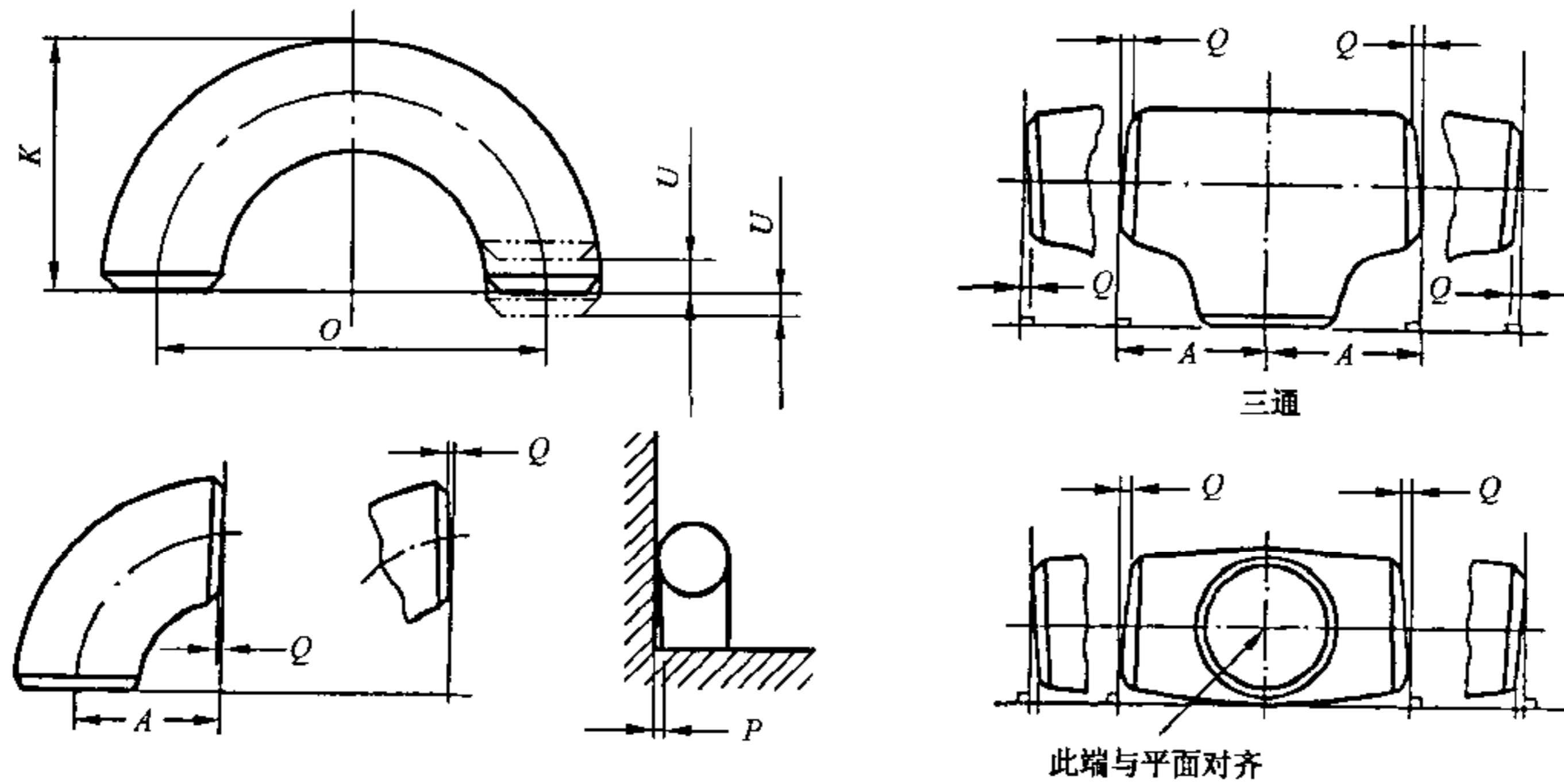
图 11 公差简图
