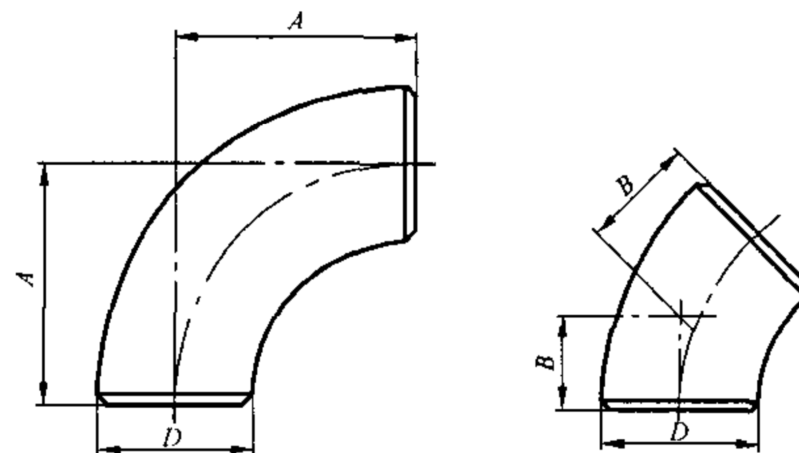
图 1 长半径弯头
