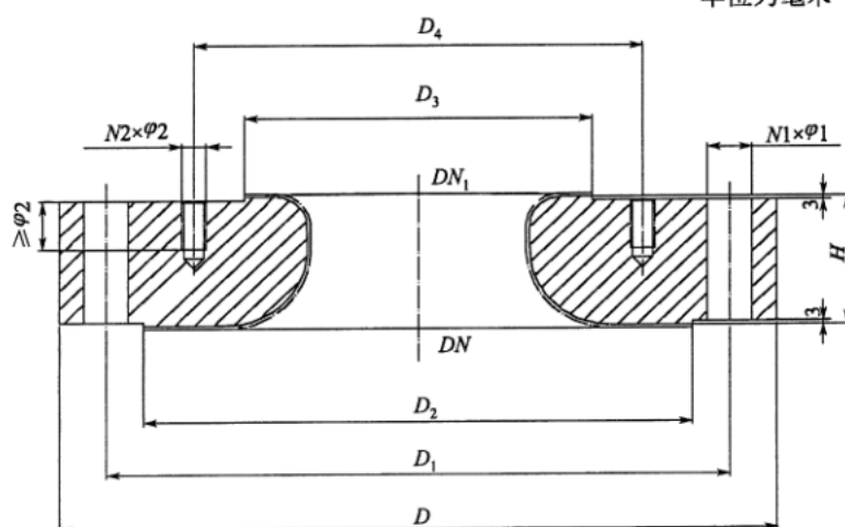
图 4 B 型搪玻璃异径法兰的型式
