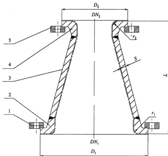
图 1 搪玻璃同心异径管的型式
