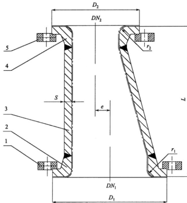
图 2 搪玻璃偏心异径管的型式
