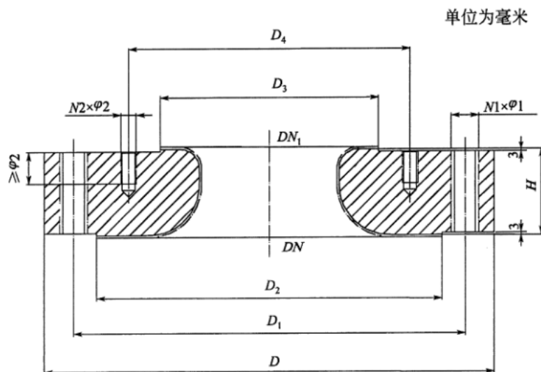
图3 A型搪玻璃异径法兰的型式
