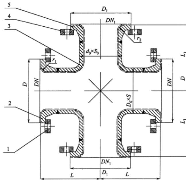
图 2 搪玻璃四通的类型
