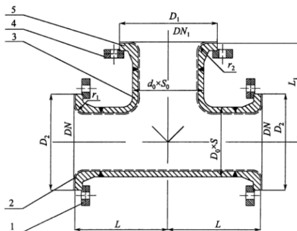
图 1 搪玻璃三通的形式
