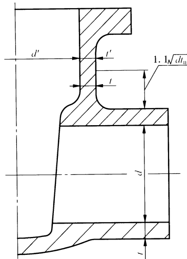
图 3 阀体颈部
