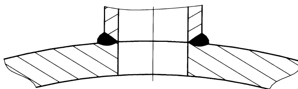
图 7 辅助连接的对焊
