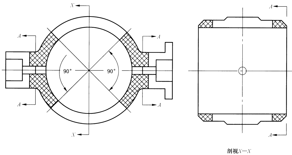
图 15 蝶阀阀体
