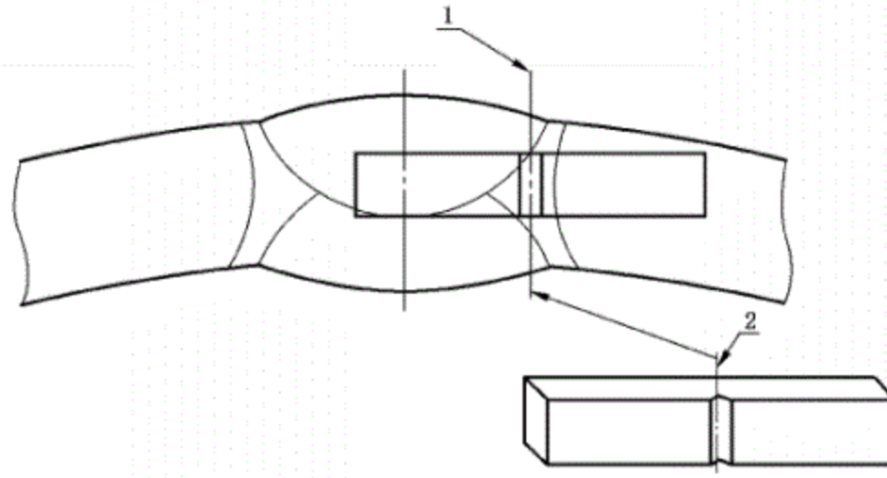
a) 热影响区试样
