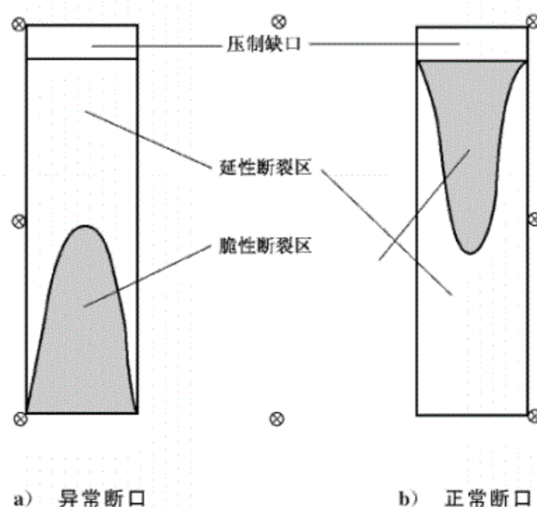
图 M.1 正常/异常典型断口示意图
