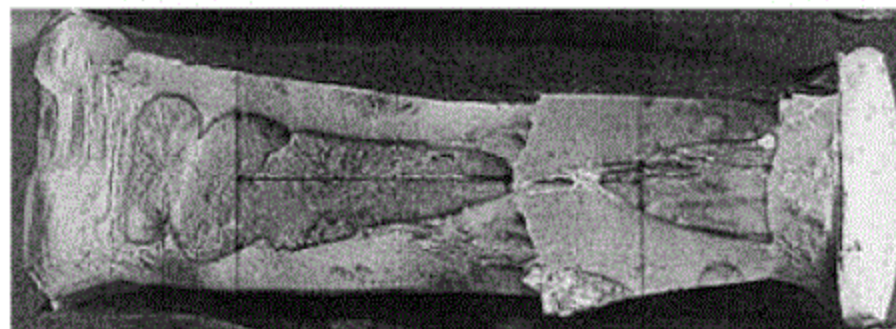
d) 第 IV 类异常断口
