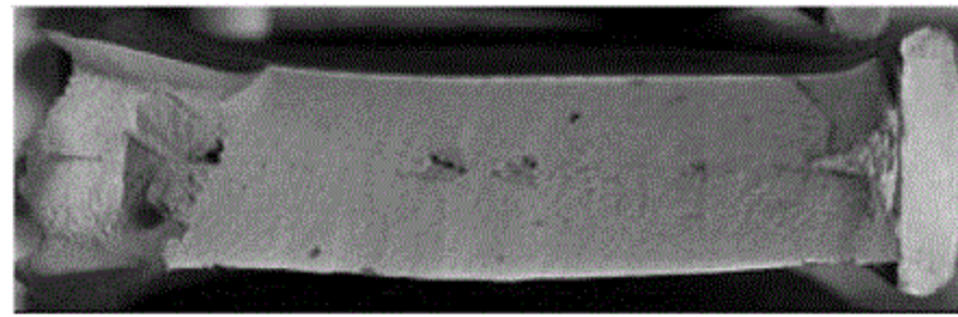
a) 第 I 类异常断口
