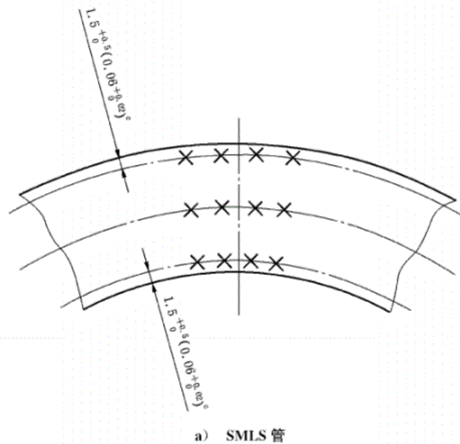
图 H.1 硬度试验位置
