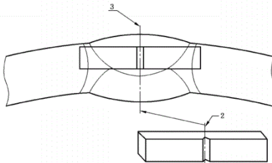
b) 焊缝试样
