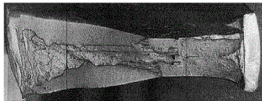
c) 第 III 类异常断口
