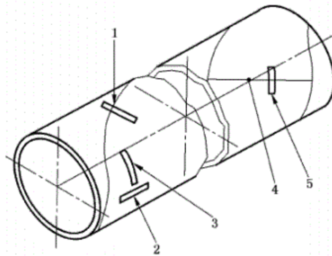
b) CW、LFW、HFW、LW、SAWL 和 COWL 管
